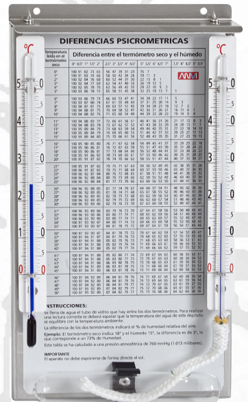
25.0635 Psicrómetro Psychrometer Psychromètre 215x120 mm
