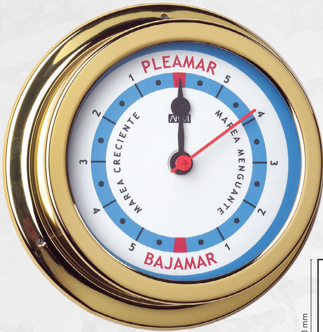
32.1126 Indicador de Mareas Tide clock Indicateur de marée
